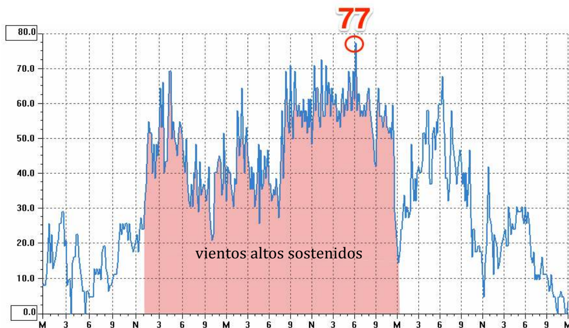
Ráfagas de viento registradas por la estación meteorológica de ALFARP entre el 19 y el 21/01/20 (en km/h)
