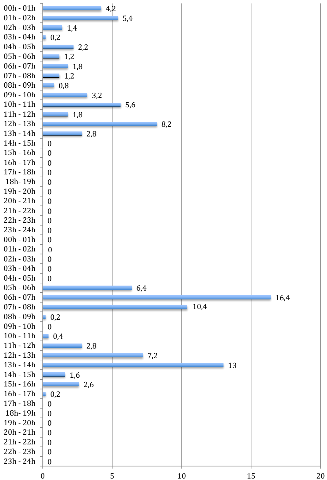
Cantidades de lluvia registradas por horas en ALFARP los días 21 y 22 de enero de 2020 (en l/m²)
